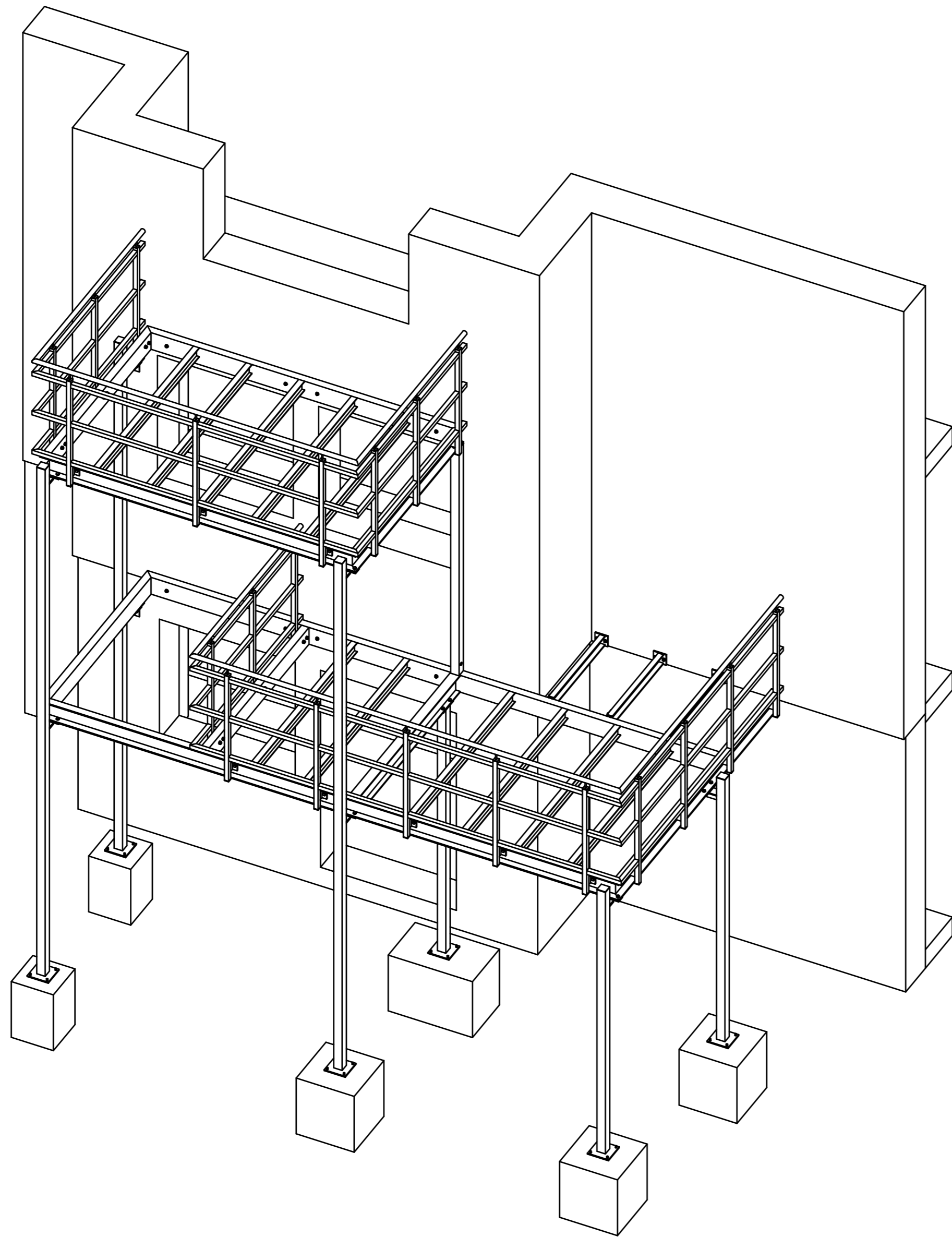
3D Übersicht
